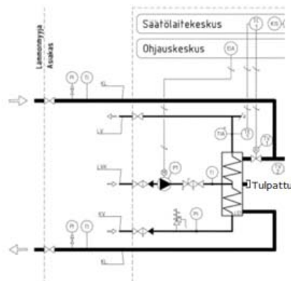
Esimerkki kytkentäkaaviosta, jossa lämmityksen lämmönsiirtimeltä palaavan putken yhde tulputtu.
